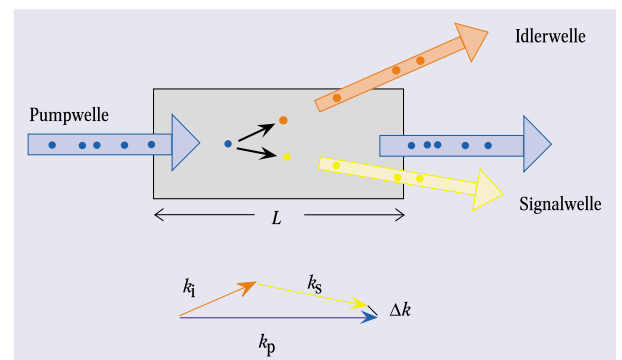
Abb. 3: Die Oszillation wird durch parametrische Fluoreszenz ausgelöst, die als Photonenpaftung veranschaulicht werden kann: Ein Pumpphoton wird vernichtet, ein Signal- und ein Idlerphoton erzeugt. Die Wahrscheinlichkeit für diesen Prozess liegt bei ca. 10^{-10} pro Pumpphoton. Es werden hauptsächlich Photonenpaare erzeugt, deren Wellenvektoren näherungsweise die Impulserhaltung \Delta k = k_p - k_s - k_i = 0 (Phasenanpassungsbedingung) erfüllen. Diese Bedingung bestimmt die Ausbreitungsrichtung von Signal- und Idlerwellen.
