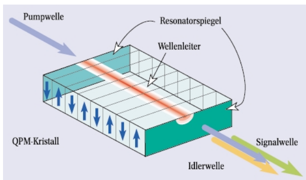
Abb. 10: In einem Wellenleiter-OPO wird das Laserlicht im nichtlinearen Kristall nah an der Oberfläche geführt. Ein solches System wurde durch Einlagerung von Titanatomen unter die Oberfläche eines \text{LiNbO}_3 -Substrats realisiert [19]. Damit geht eine Variation des Brechungsindex einher, die das Laserlicht unter der Oberfläche führt. Als Resonatorspiegel dienen dielektrische Schichten auf den Kristalloberflächen, als Pumpquelle ein abstimmbarer Diodenlaser, der eine weite und schnelle Abstimmung der Signalwellenlänge ermöglicht.
