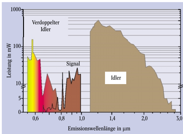
Abb. 9: Mit einem Festkörperlaser-gepumpten SRO, speziell in Multigitterkristallen, und anschließender Frequenzverdopplung erzielt man einen breiten Emissionsbereich. Bis auf eine Lücke um 1064\ \text{nm} (doppelte Pumpwellenlänge) wird der gesamte Spektralbereich von 560\ \text{nm} bis 2670\ \text{nm} abgedeckt [10].
